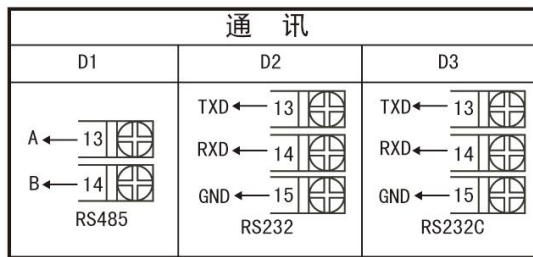
图 6 A、B 型统一变送接线图
