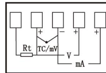
通道输入 5
