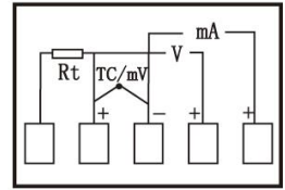
通道输入 1
