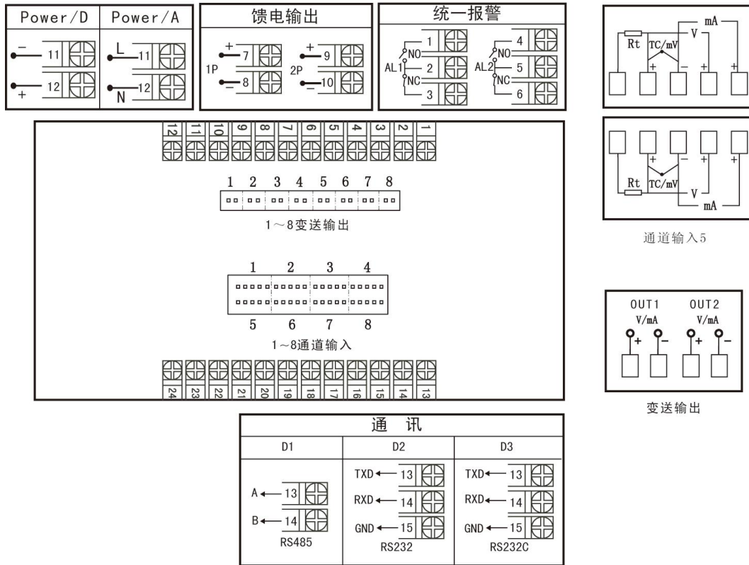
图 10 C 型分别变送接线图
