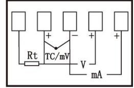
通道输入 5
