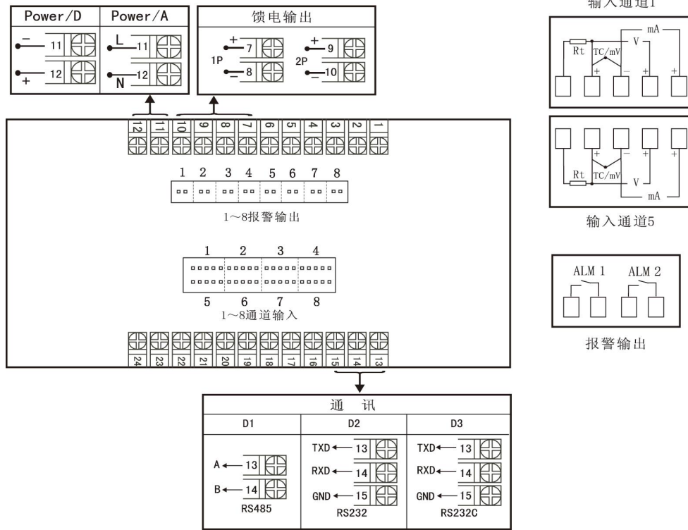
图 6 C 型分别报警接线图
