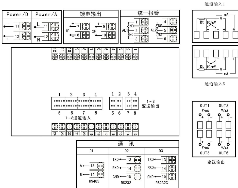
图 5 A、B 型分别变送接线图
