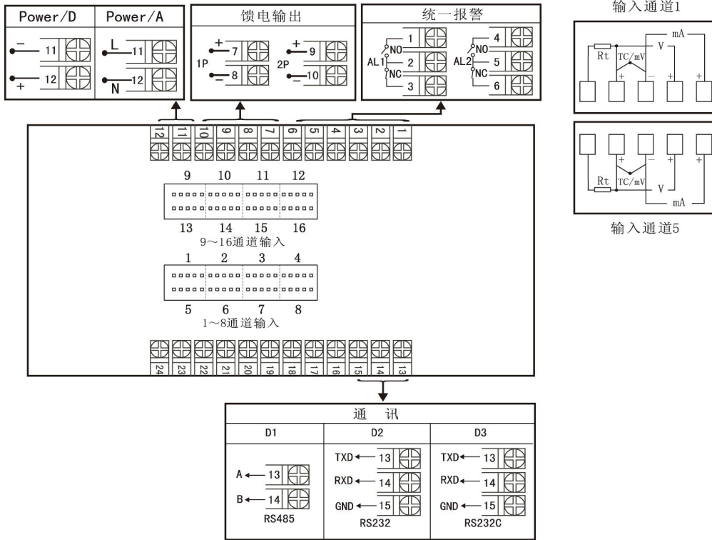
图 2 A、B、C 型统一报警接线图
