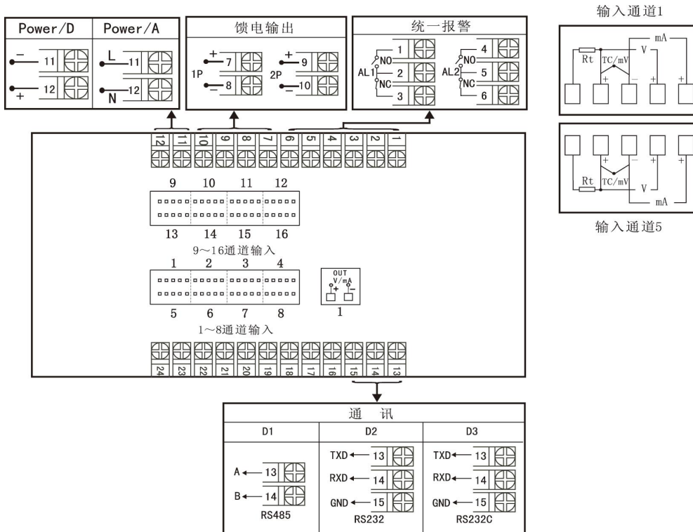
图 3 A、B 型统一变送接线图
